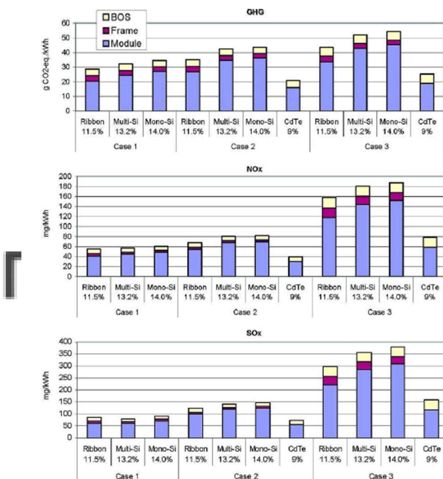
Εικόνα 7.10: Ανάλυση αέριων εκπομπών κύκλου ζωής ενός ΦΒ συστήματος
