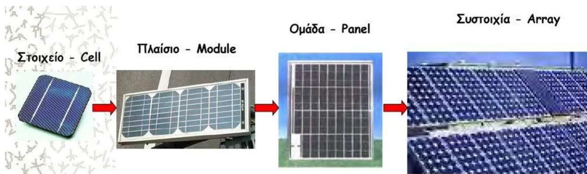
Εικόνα 7.4: Φωτοβολταϊκή συστοιχία
