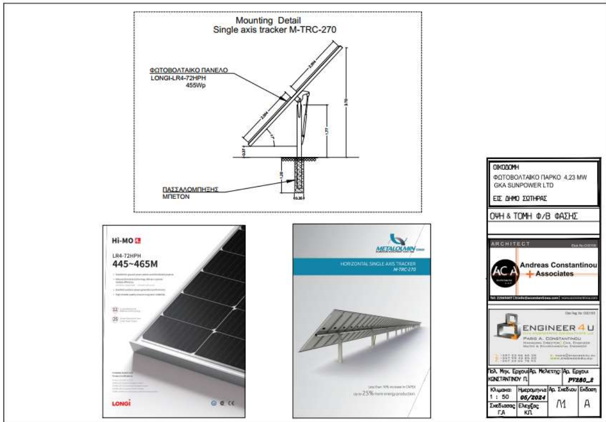
Εικόνα 7.5: Έδραση πλαισίων, βάση ιχνολατ
