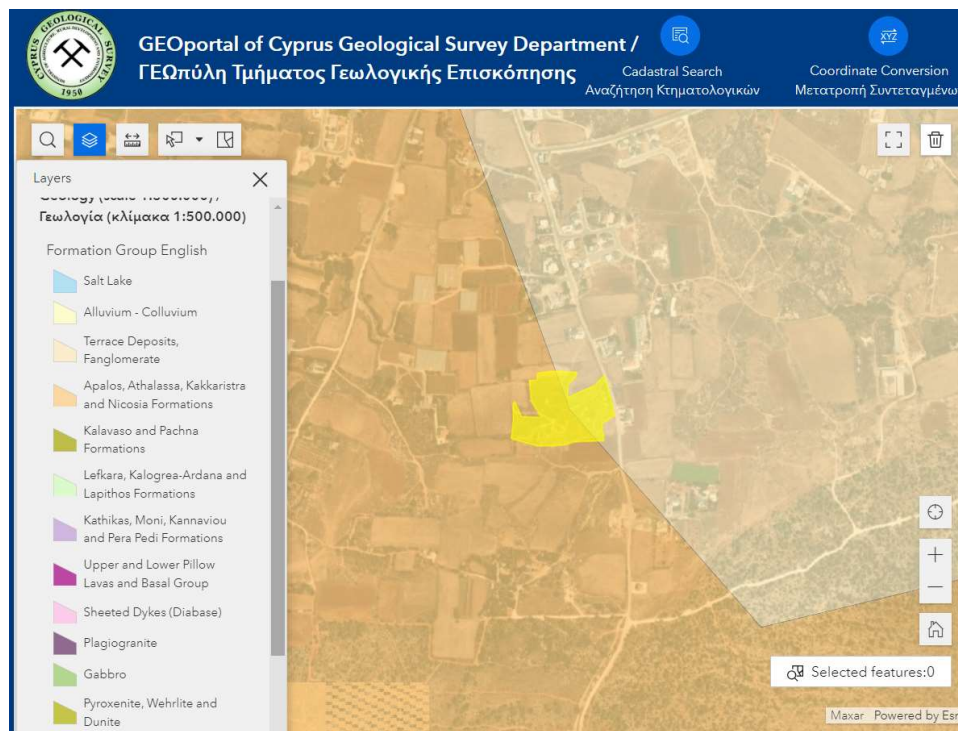
Εικόνα 6: Γεωλογικοί σχηματισμοί
