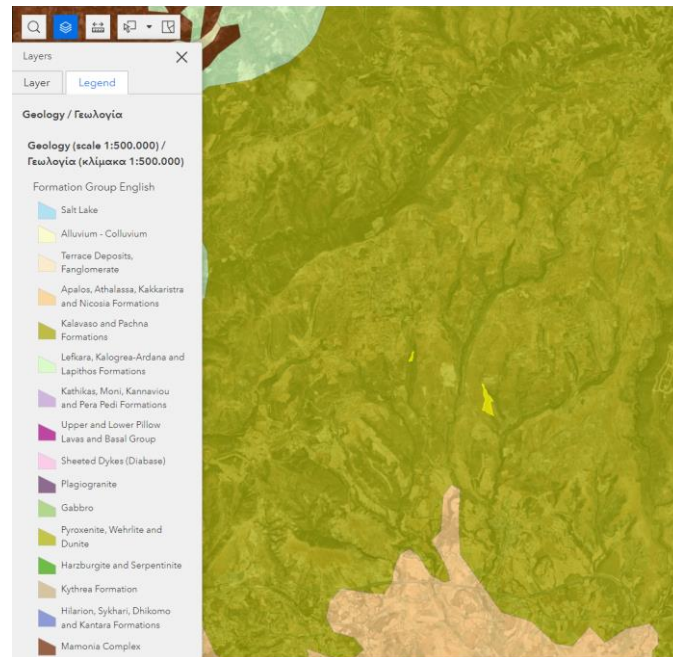
Εικόνα 6: Γεωλογικοί σχηματισμοί
